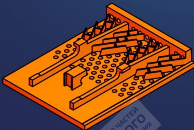
Колосник VL (поз. 896) СЛ-2546002-964В1 Сталь 35Х23Н7СЛ
