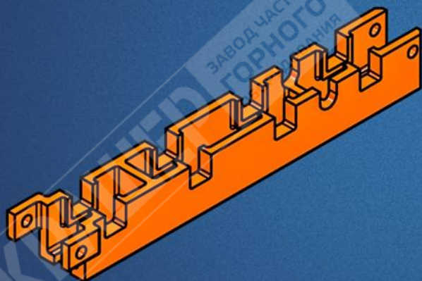
Путь роликовый II средний РЕКАТ-...(L2-14425)17-003 Сталь 20Х25Н19С2Л
